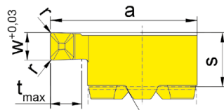
Klemhalter Stirnseite Toolholder face
