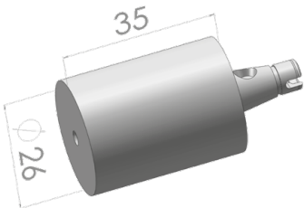
Drehhalter Rohling \varnothing 26 Turning holder blank \varnothing 26
