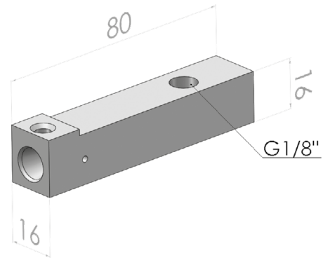
Statischer Halter 16x16VKT mit IKZ Static holder with internal cooling Bestellnummer WFMS.VKT.016.IK Order no.
