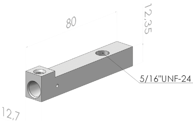
Statischer Halter 12,7x12,7VKT mit IKZ Static holder with internal cooling Bestellnummer WFMS.VKT.012,7.IK Order no.
