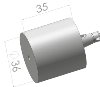
Drehhalter Rohling \varnothing 36 Turning holder blank \varnothing 36
